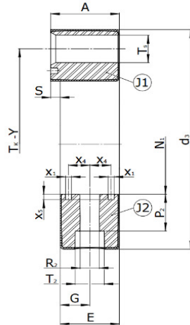
Size 001, 002
